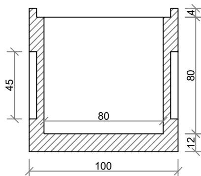
Pozzetto: sezione A-A
