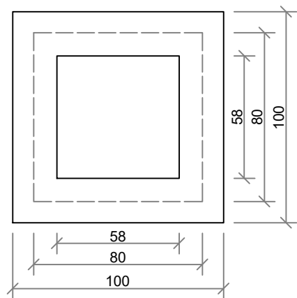
Chiusino - vista in pianta
