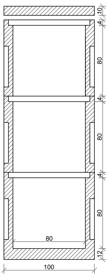
ASSEMBLAGGIO TIPO (con prolunghe) vista in sezione
