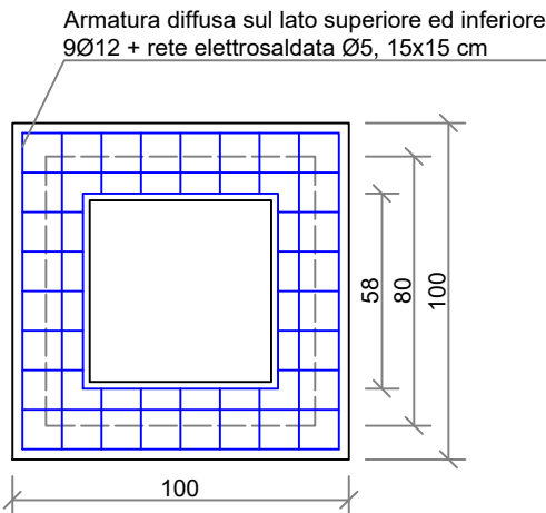
ARMATURA DEL COPERCHIO
