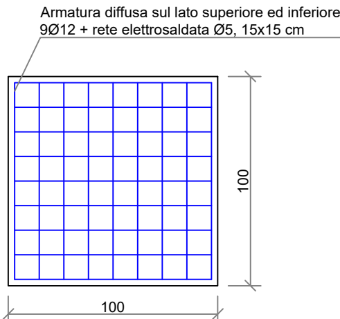
ARMATURA PLATEA
