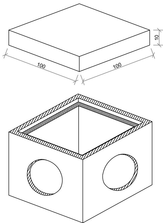
Vista assonometrica
