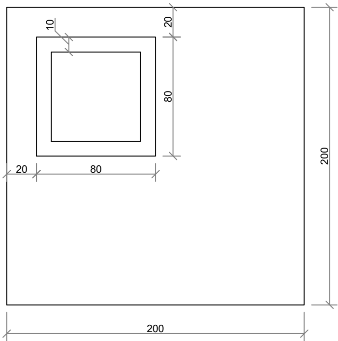
Chiusino - vista in pianta
