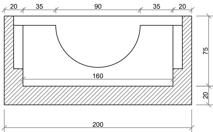
Pozzetto: sezione A-A
