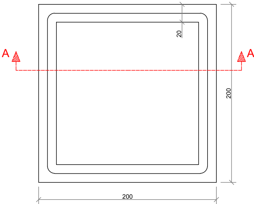
Pozzetto - vista in pianta
