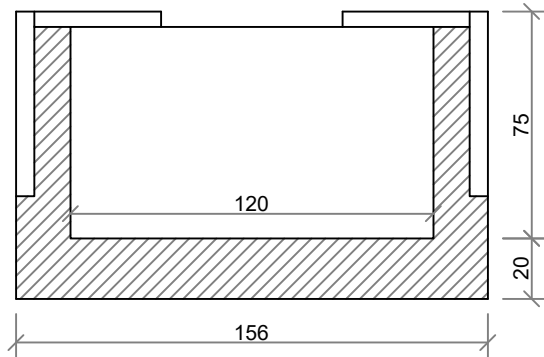
Pozzetto: sezione A-A
