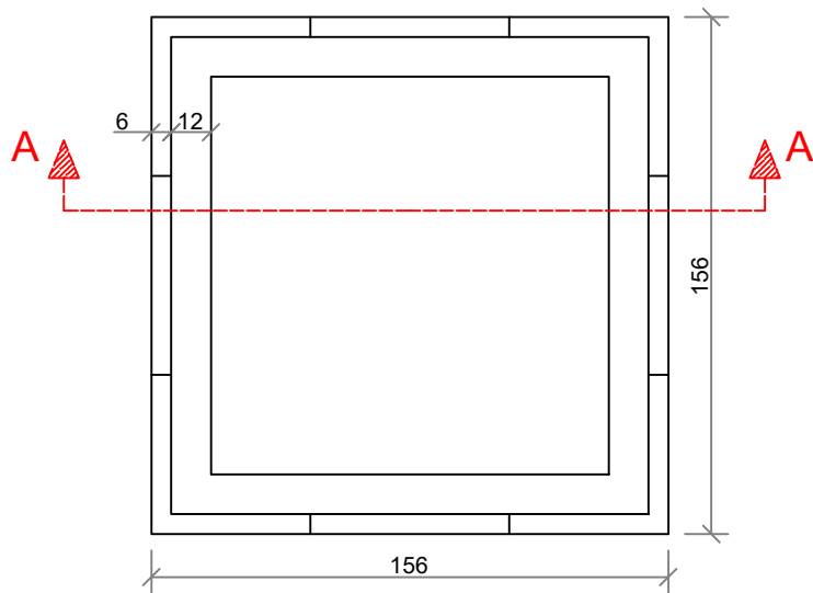
Pozzetto - vista in pianta
