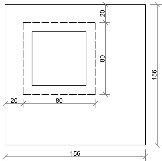
Chiusino - vista in pianta
