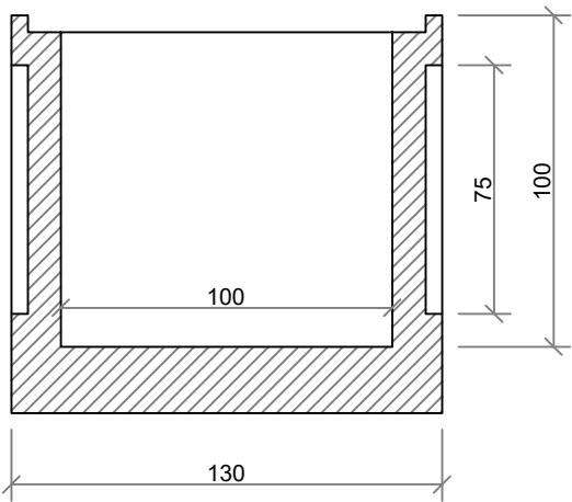
Vista in sezione
